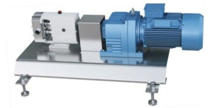
Bomba Sanitaria de Desplazamiento Positivo DIISA Modelo Lobular DUL 30 2"
